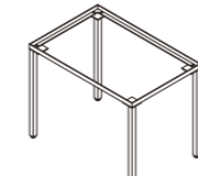
(b)-2脚フレーム H:700 W:900 D:600 クロームメッキ
