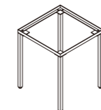
(a)-2脚フレーム H:700 W:600 D:600 クロームメッキ
