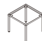
(a)-1脚フレーム H:500 W:600 D:600 クロームメッキ
