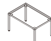
(b)-1脚フレーム H:500 W:900 D:600 クロームメッキ
