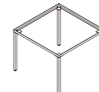
(e)脚フレーム H:700 W:900 D:900 クロームメッキ
