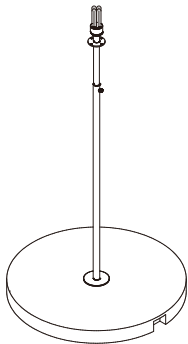
(a)フロアースタンド H:1685~2435 φ:1050 ステージ:メラミン化粧板 支柱:クロームヘアライン ランプ付
