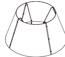
(c)-2円錐型セード(大) H:436 上辺:φ750 下辺:φ1150 フレーム:メラミン焼付塗装(白全艶) セード:ポリプロピレン
