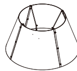
(c)-1円錐型セード(小) H:436 上辺:φ550 下辺:φ850 フレーム:メラミン焼付塗装(白全艶) セード:ポリプロピレン
