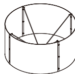
(d)-1円柱型セード(小) H:436 φ:850 フレーム:メラミン焼付塗装(白全艶) セード:ポリプロピレン
